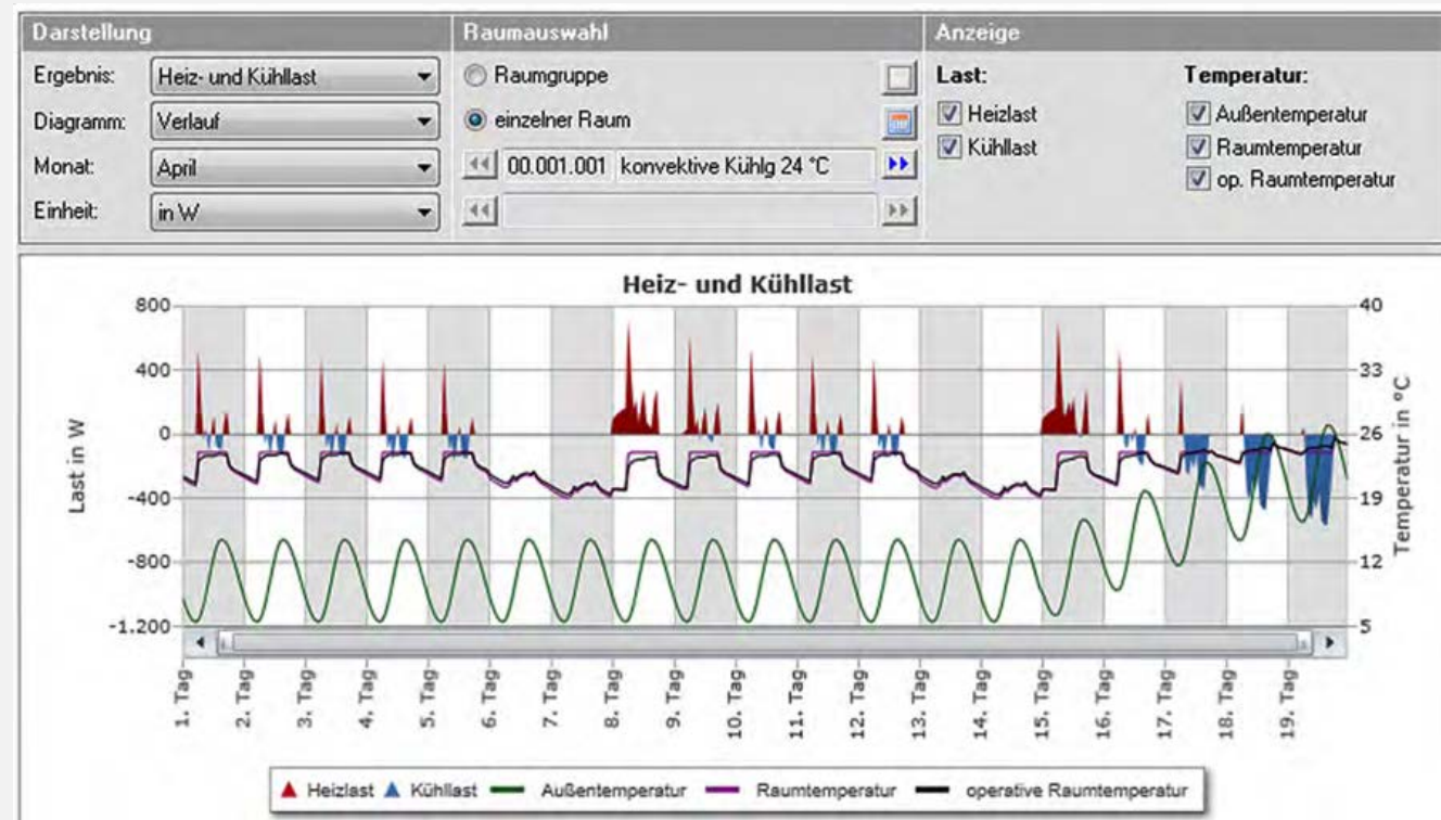
Abb. 13 Stündliche Werte der Jahressimulation der Heiz- und Kühlenergie sowie der Außentemperatur.
