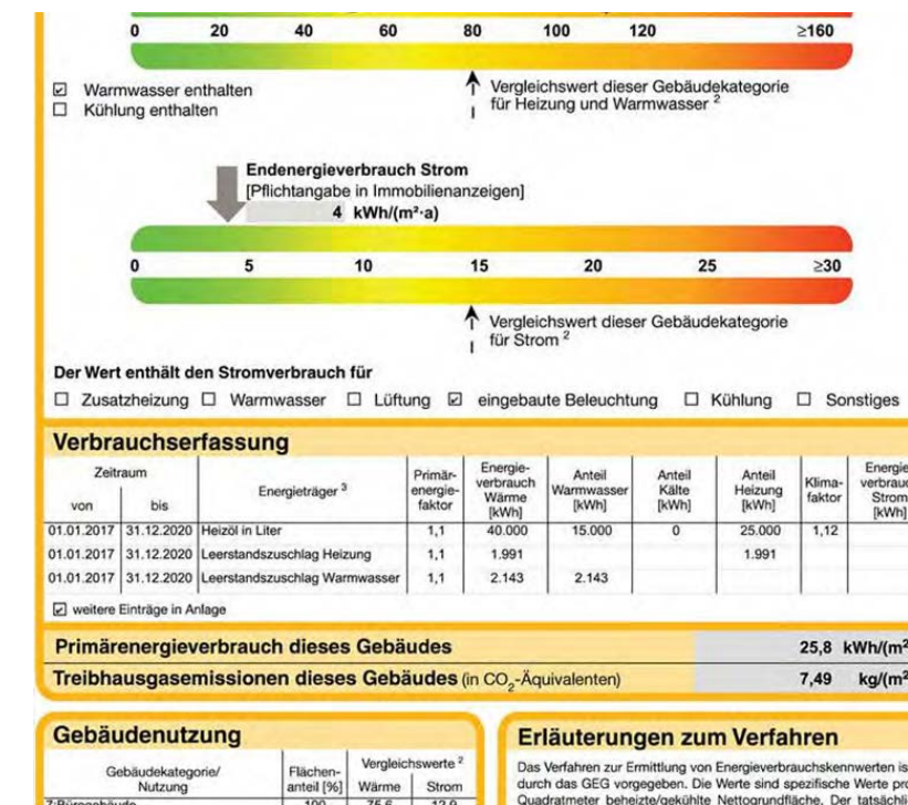
Abb. 25 Verbrauchsausweis (Auszug) nach GEG für ein Wohn- oder Nichtwohngebäude inkl. Nachweis der Treibhausgasemission (CO 2 -Äquivalent)
