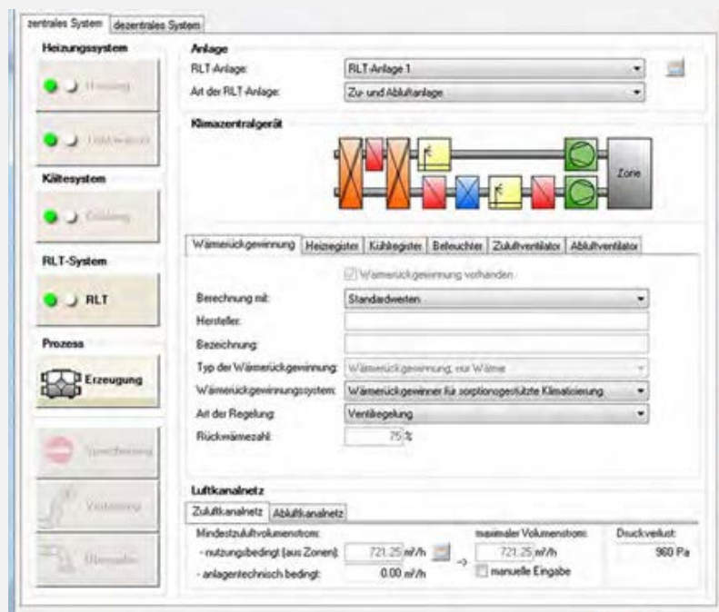
Abb. 22 Dialog zur Datenbearbeitung des Wärme-/Kälte-Erzeugers nach DIN V 18599 für ein Nicht-Wohngebäude im Rahmen der Nachweis-Erstellung nach GEG.
