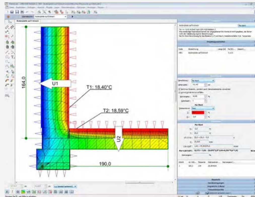
Abb. 3 Dialog zum Berechnen einer 2D-Wärmebrücke (Bodenplatte gegen Erdreich). Darstellung der Wärmebrücke mit Isothermen, FEM-Gitter und Temperaturen an ausgewählten Oberflächen-Punkten.
